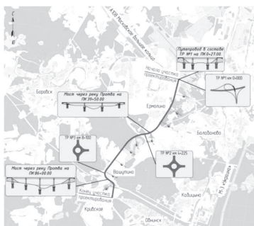
Автомобильная дорога «Обход города Балабаново»
