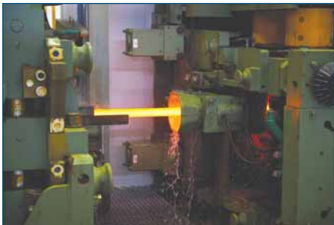
Заготовка в прокатном цехе
