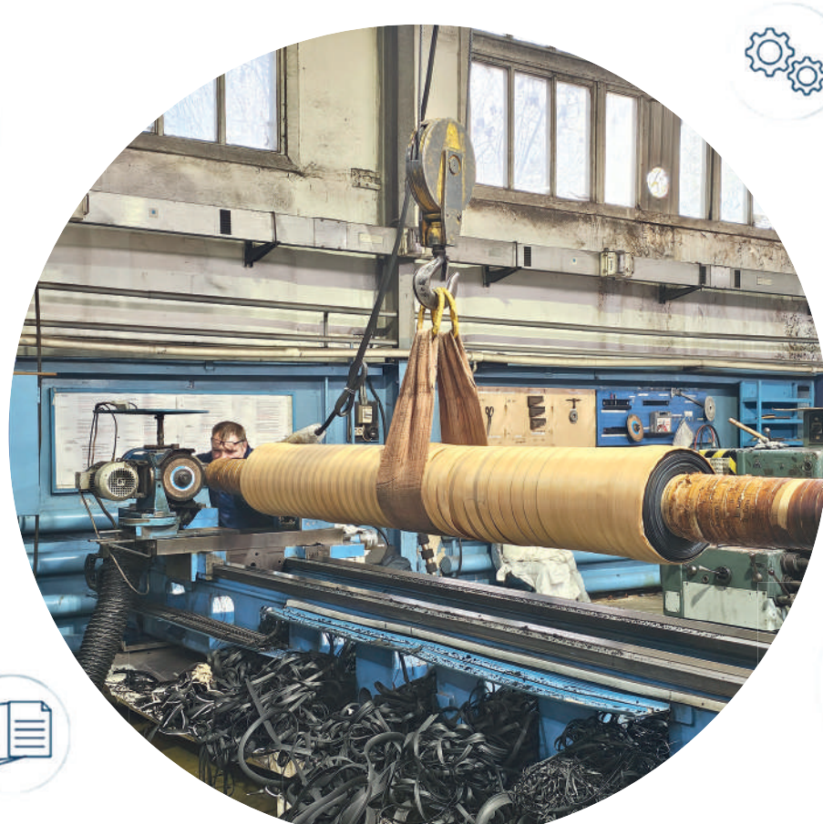
На этом станке производится предварительная шлифовка ролика
